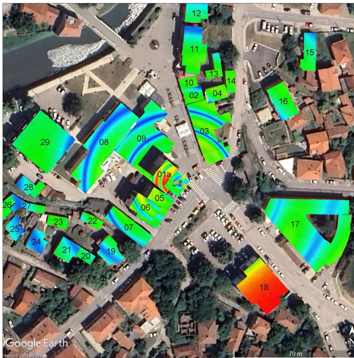
Слика 4.11. Јачина електричног поља унутар објекта када радио-систем LTE1800 оператора Telekom Srbija ради максималним капацитетом
