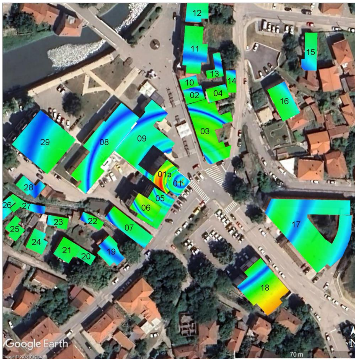
Слика 4.12. Јачина електричног поља унутар објекта када радио-систем LTE2100 оператора Telekom Srbija ради максималним капацитетом
