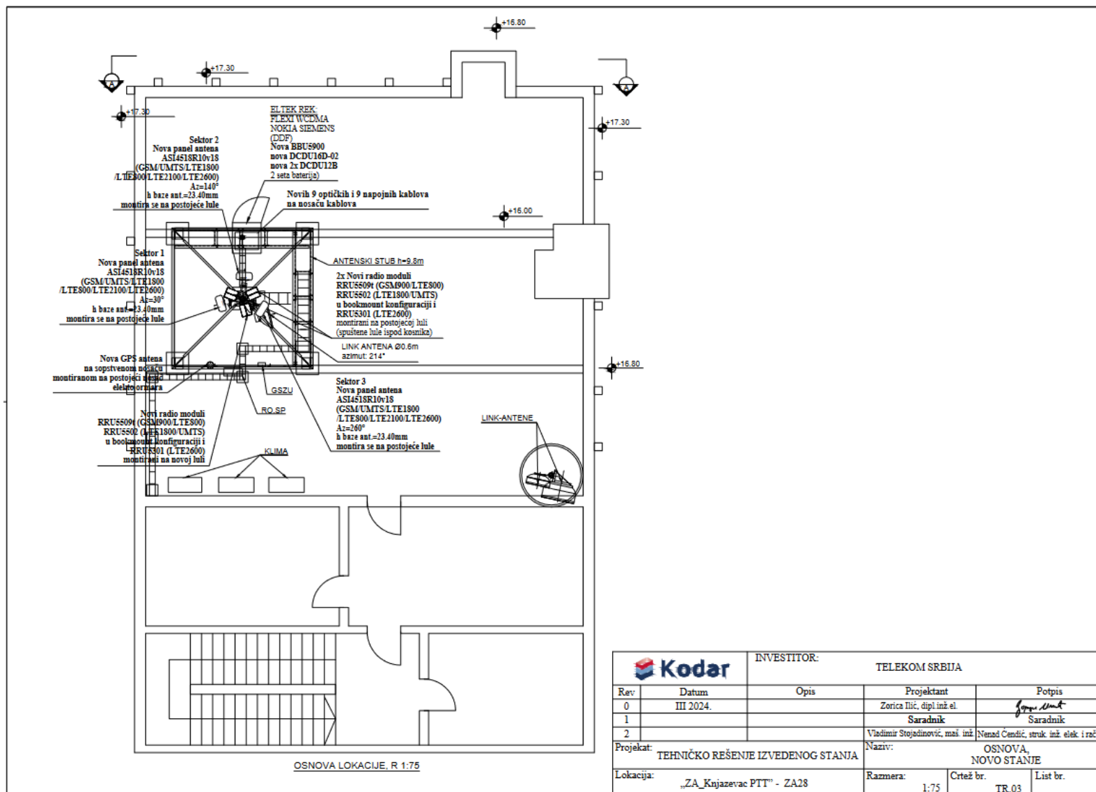
Слика 8.1. Диспозиција опреме на локацији – основа локације
